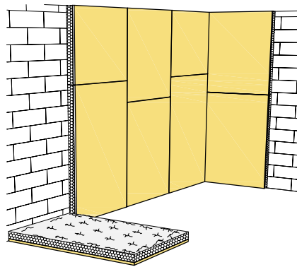
Dünnbettverfahren bei ebenem Untergrund.
