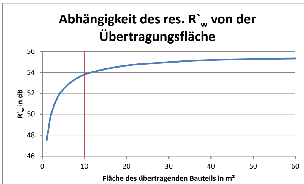
Abbildung 16: Darstellung des sich einstellenden resultierenden Luftschalldämm-Maßes bei Flächen kleiner 10 \text{ m}^2 für das Beispiel aus dem Massivbau
