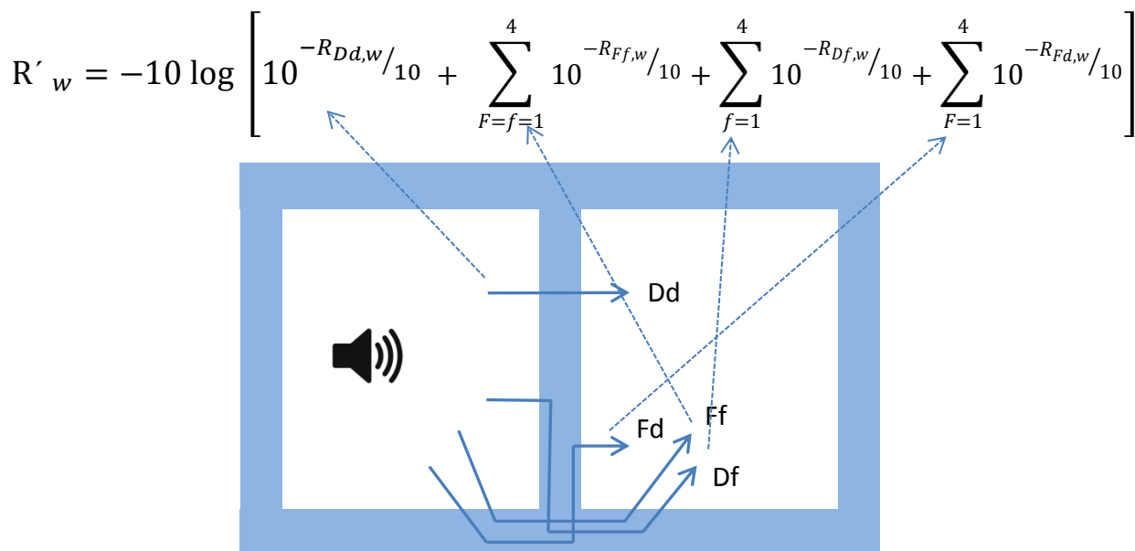
Abbildung 3: Zusammenstellung der möglichen Schallübertragungswege nach DIN 4109-2:2016
