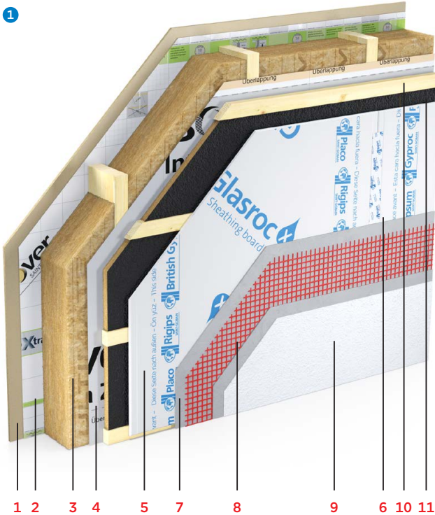
Gezeigt wird hier eine gedämmt Variante
