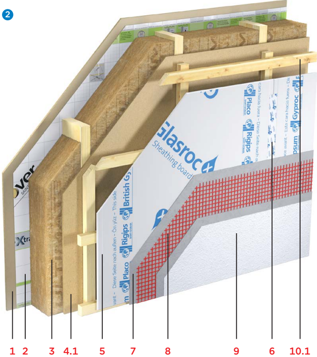
Gezeigt wird eine hinterlüftete Variante mit der Holz-Unterkonstruktion auf Holzwerkstoffplatte
